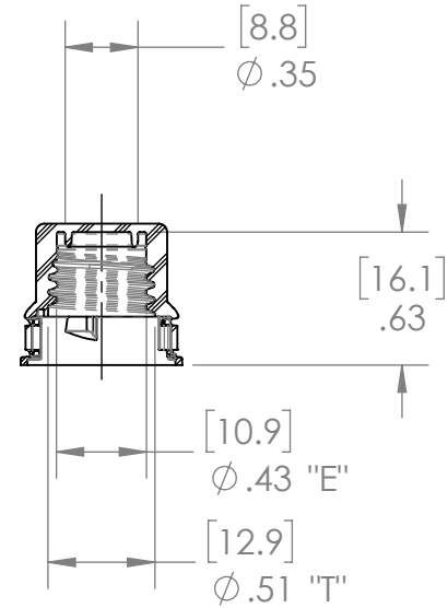
SECTION A-A
